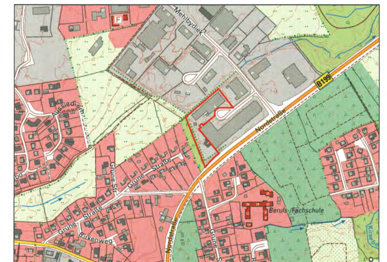
Übersichtsplan M 1:5 000
